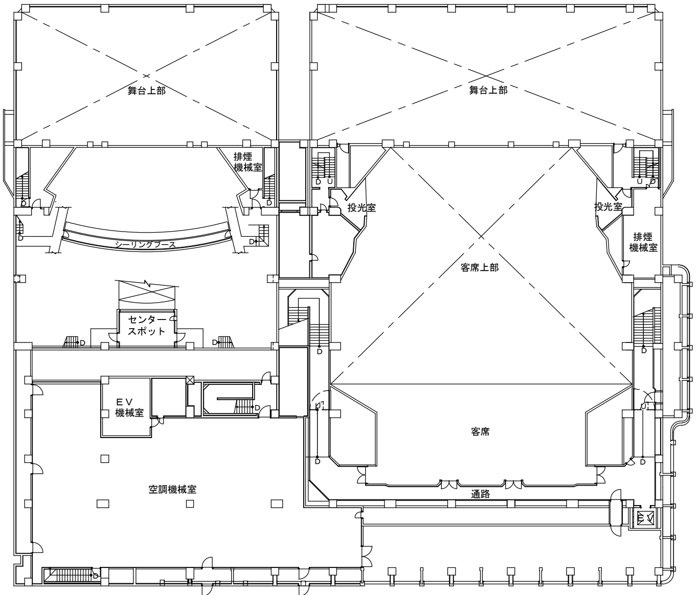
4 階 平 面 図
