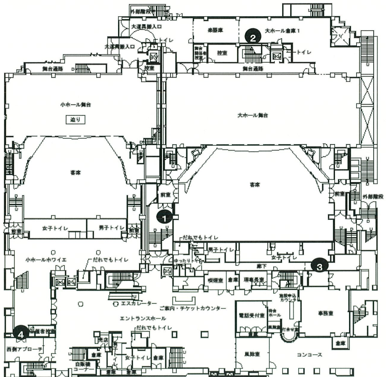
1 階平面図
